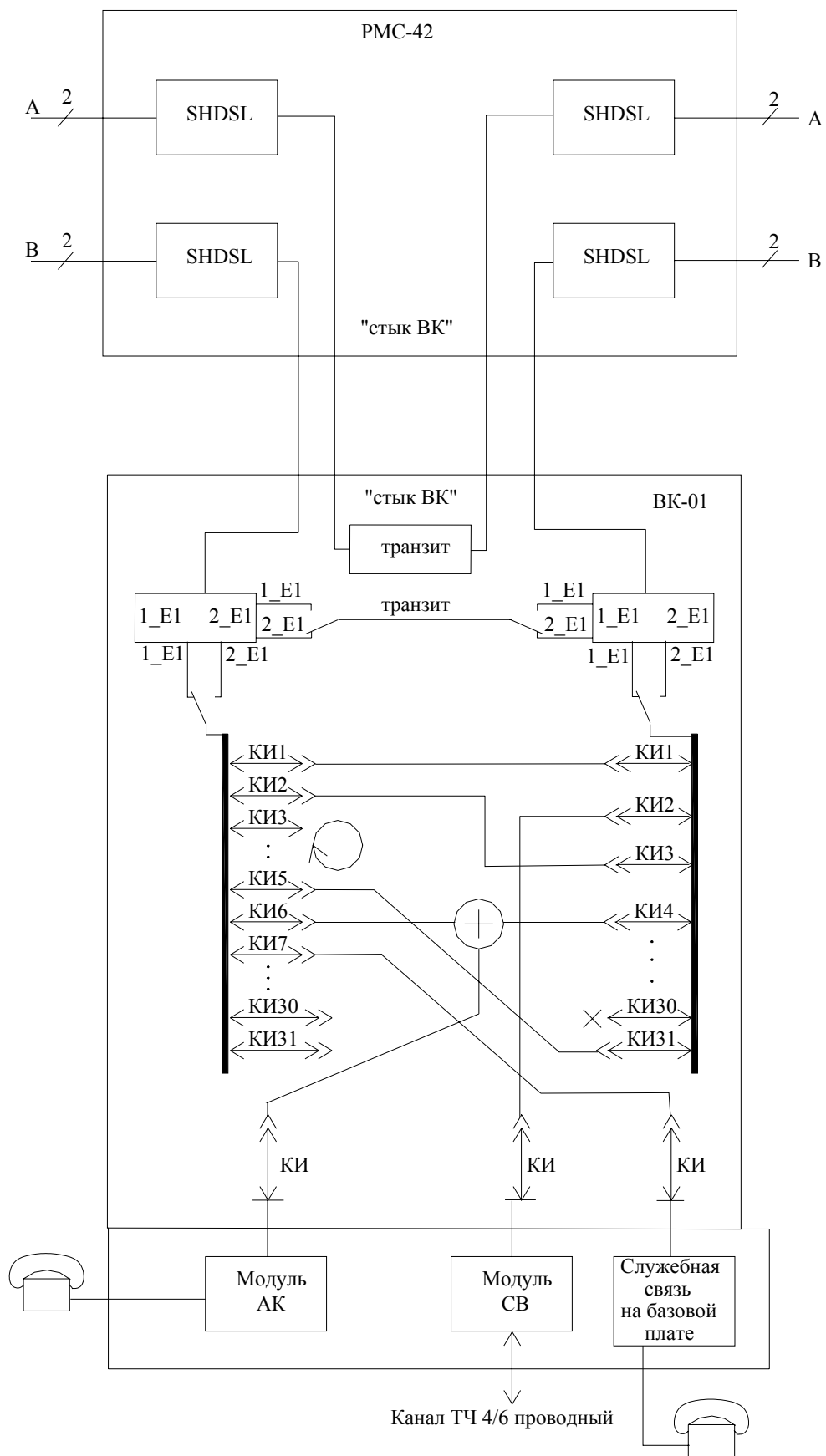
Рисунок 2 - Принцип выделения каналов из линейного сигнала
