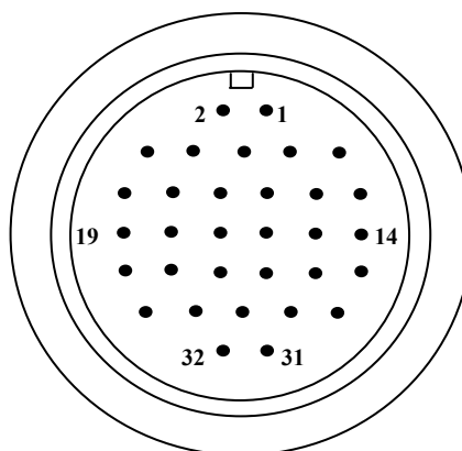
Рисунок 4 – Нумерация контактов разъёма «КО» (розетка 2РМ30КПН32Г1В1 из комплекта монтажных частей) со стороны монтажа
